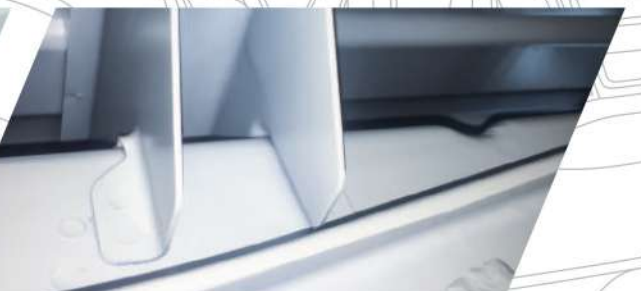
Frame kendaraan yang diperkuat; Crossbeam dengan Distribusi Daya Lebih Balanced dan kapasitas yang besar
